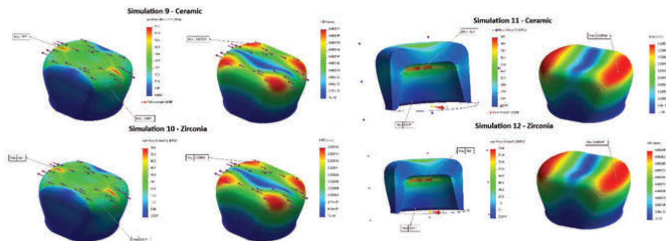
Figura 9. Rezultatet e Simulimit 9, 10, 11 dhe 12 – Stresi dhe deformim Figure 9. Results of Simulation 9,10,11 and 12 – Stress and displacement
